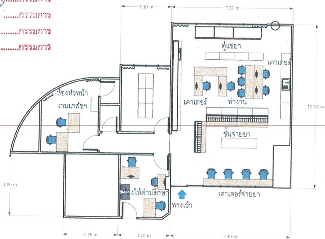
แบบแปลนงานปรับปรุงห้องจ่ายยา
